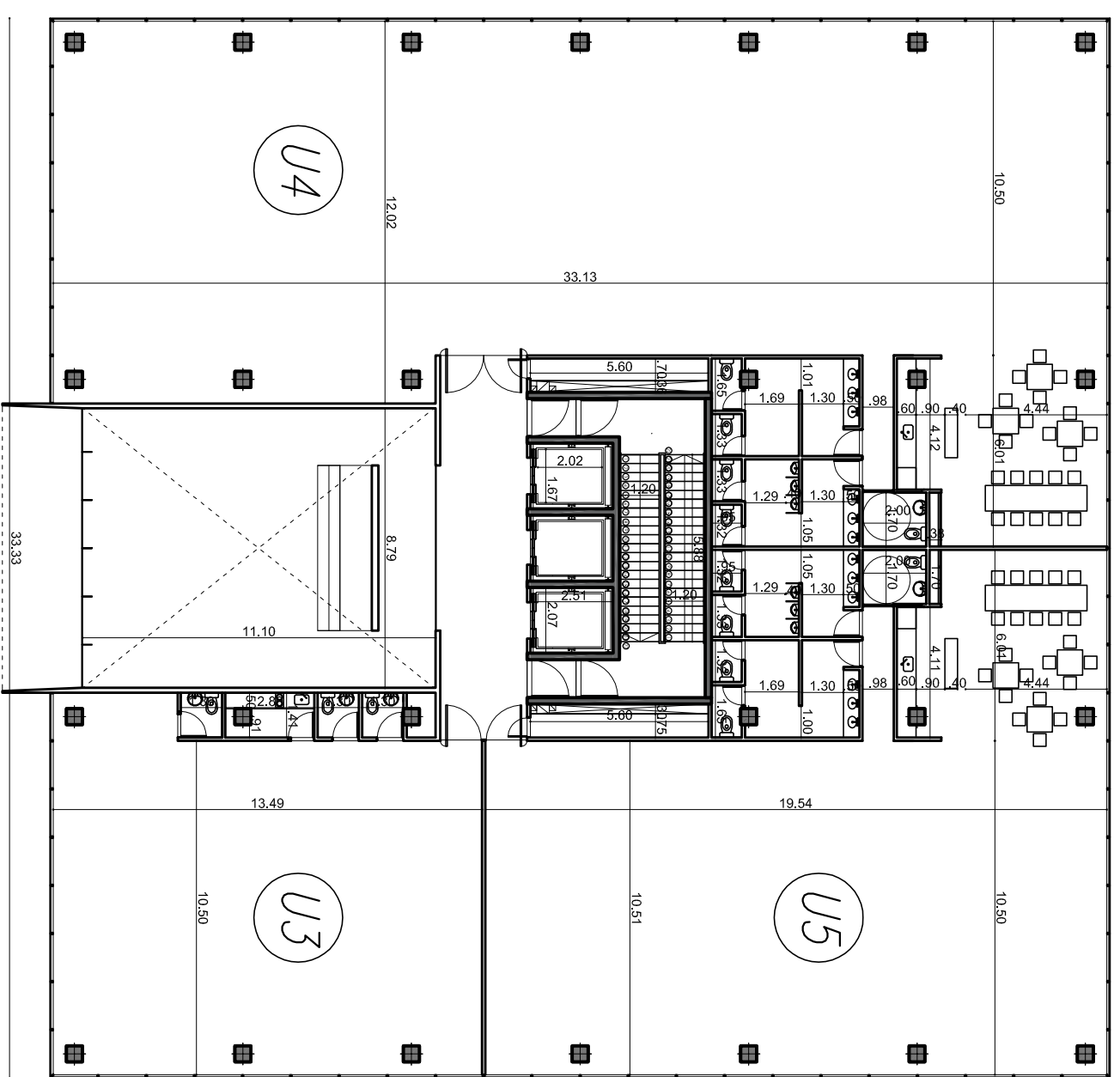
PLANTA 1° PISO
