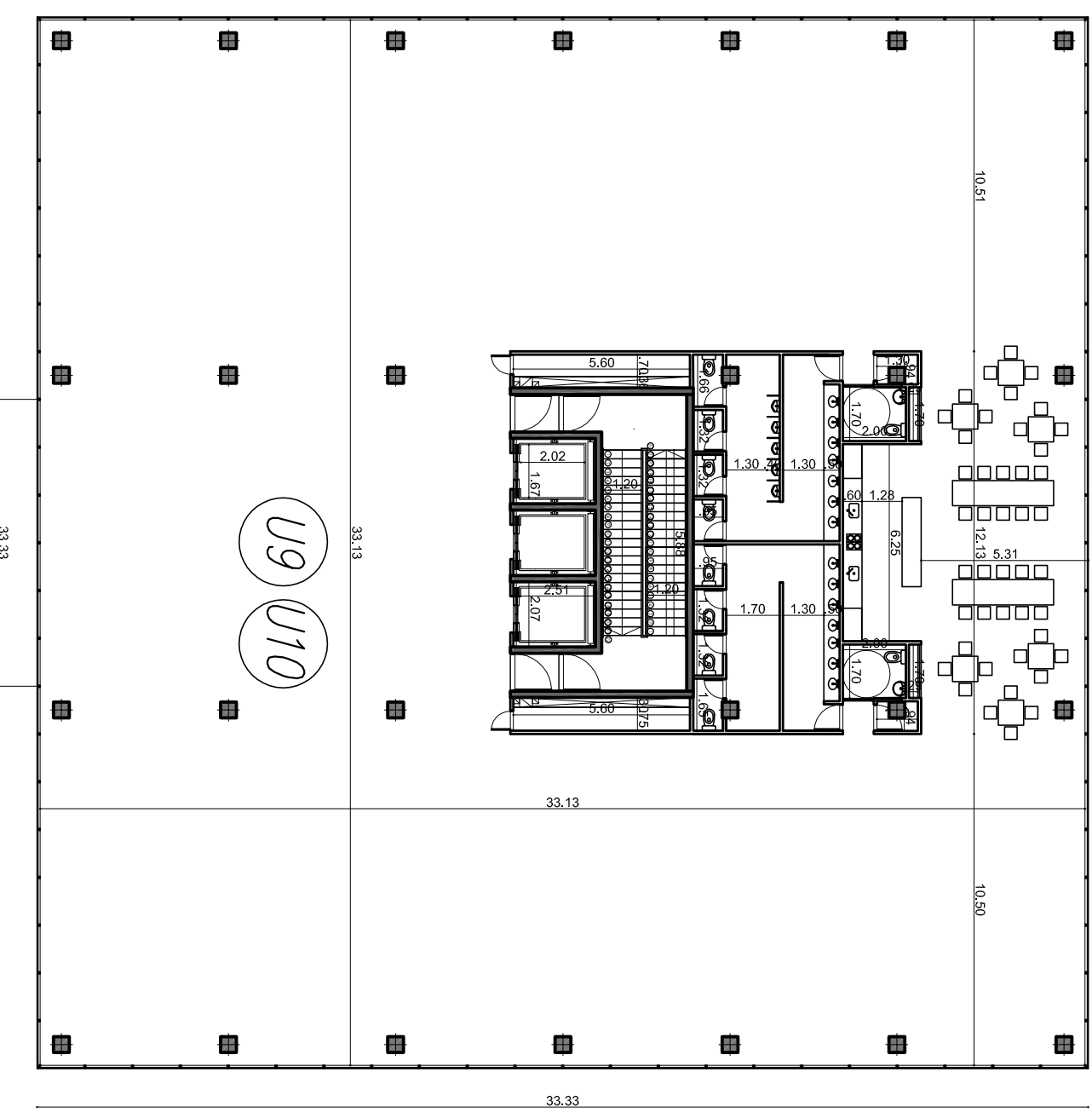
PLANTA 7° PISO
