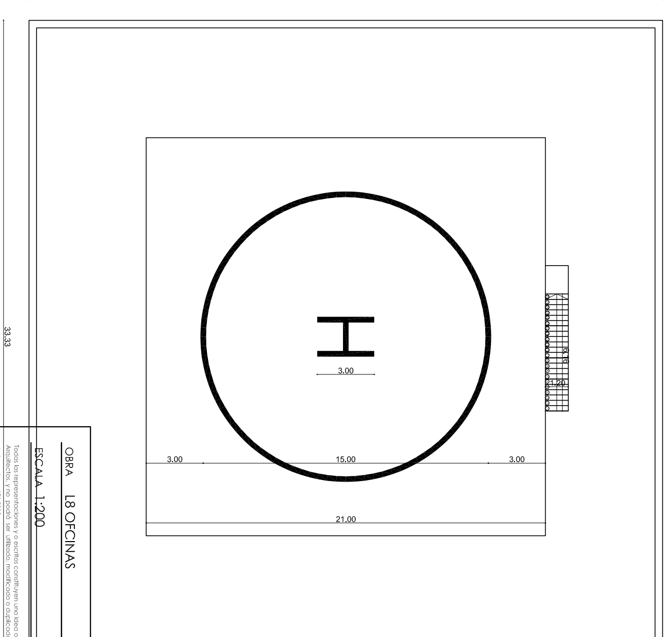
PLANTA TECHOS
