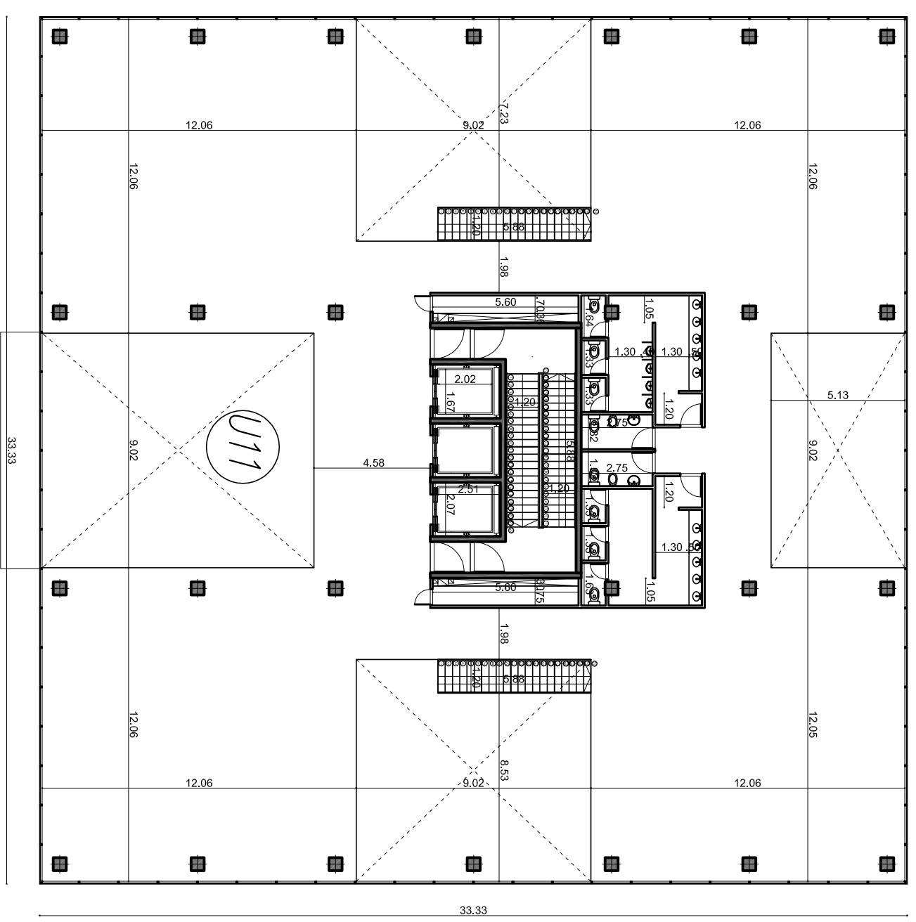
PLANTA 7° PISO
