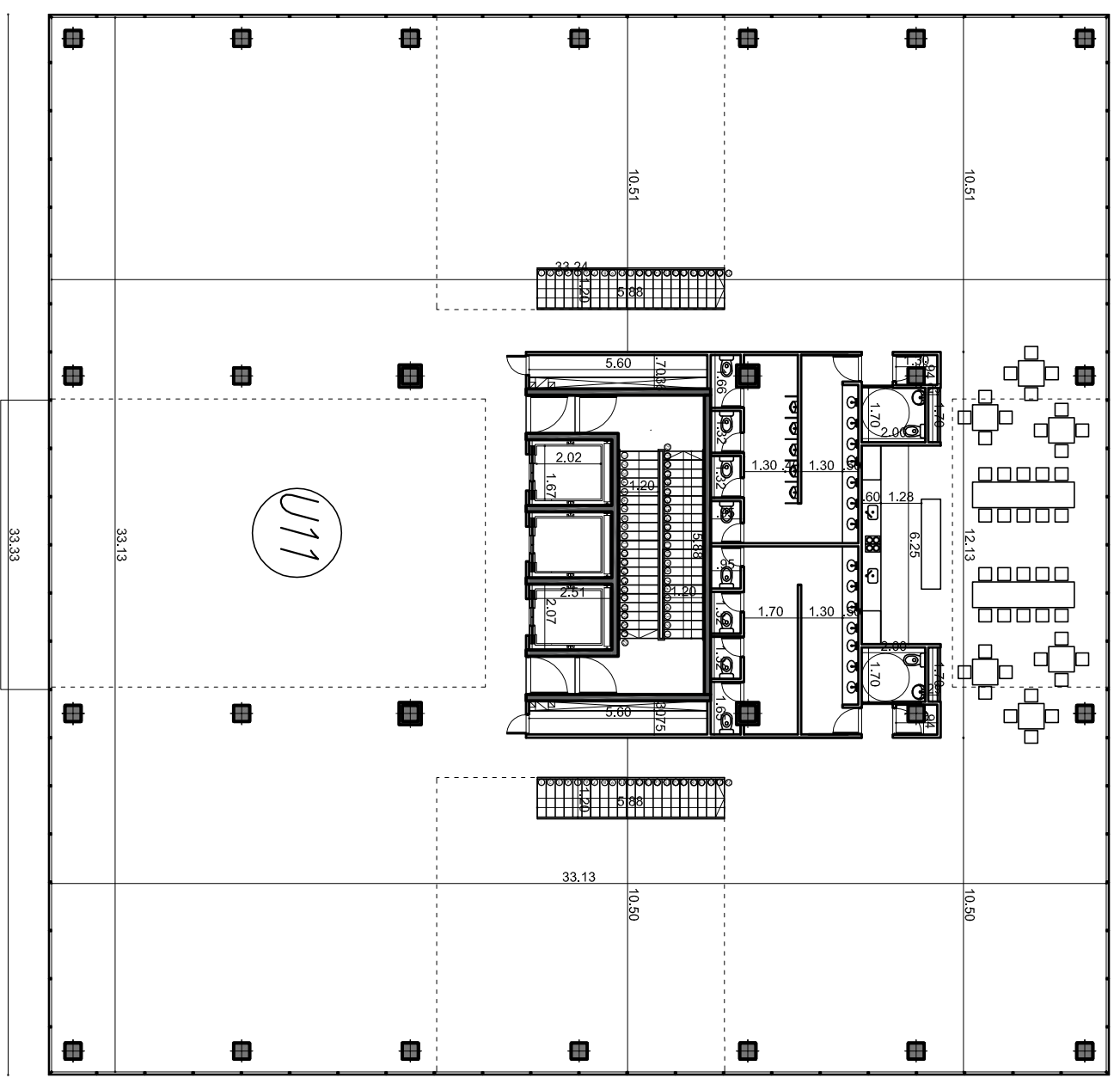
PLANTA 6° PISO
