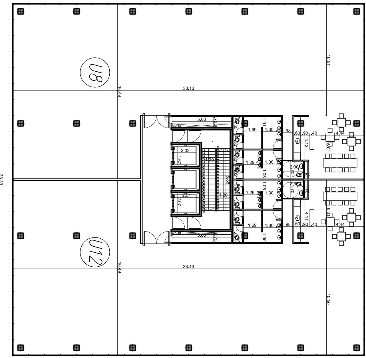
PLANTA 6° PISO
