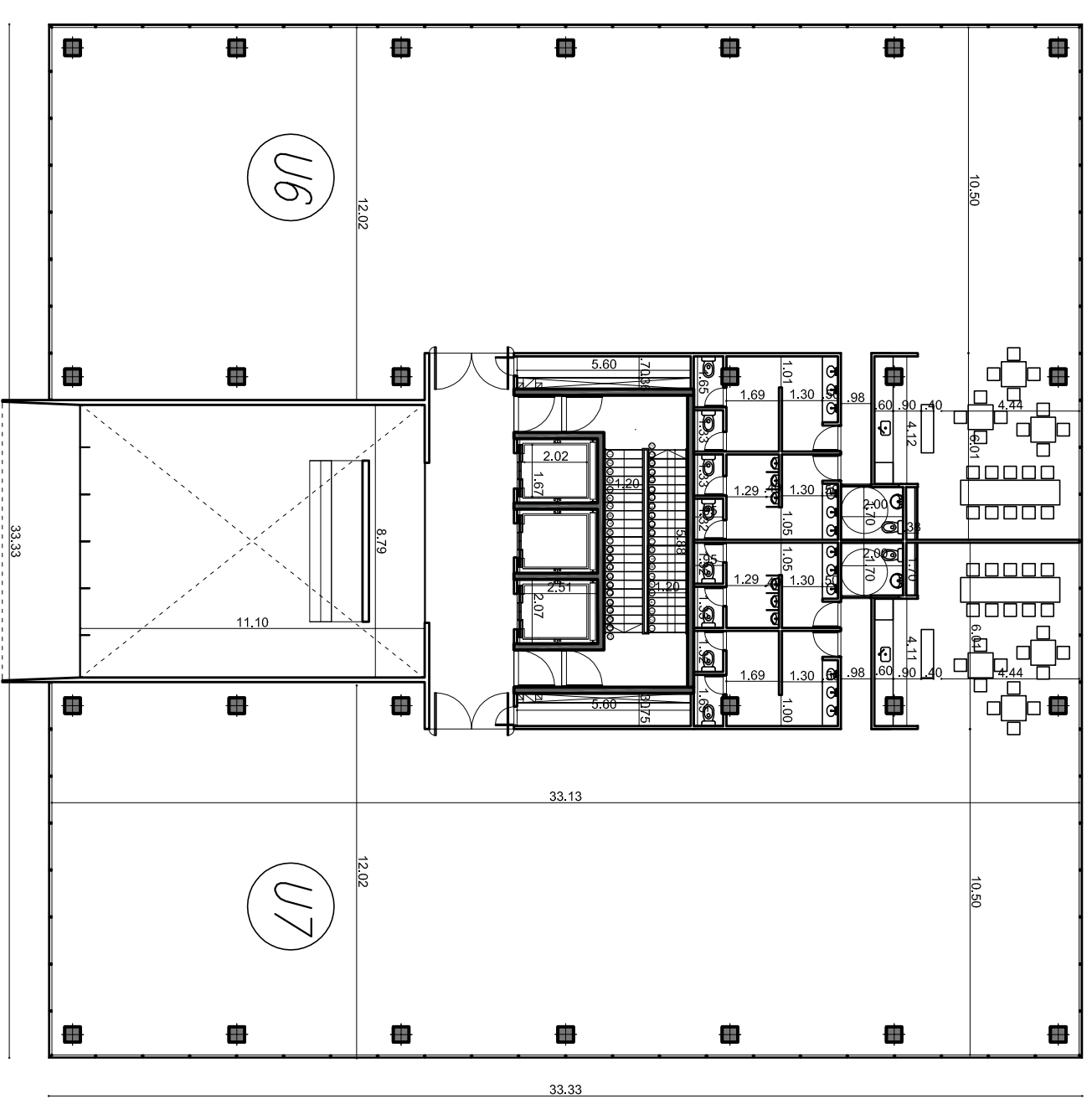
PLANTA 2° PISO
